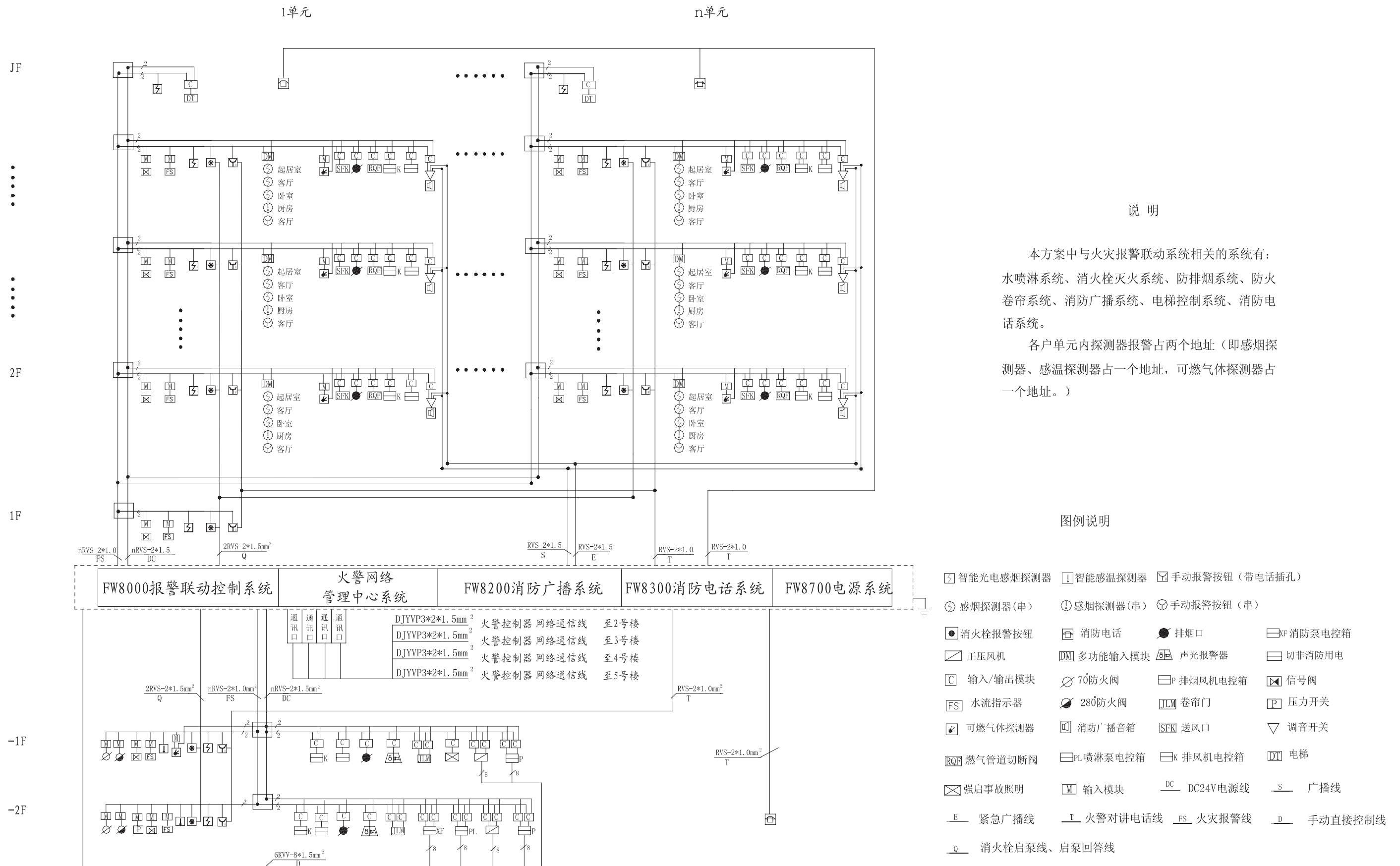
<图三>：FW8000 系统应用于高层公寓、高级住宅的系统设计
